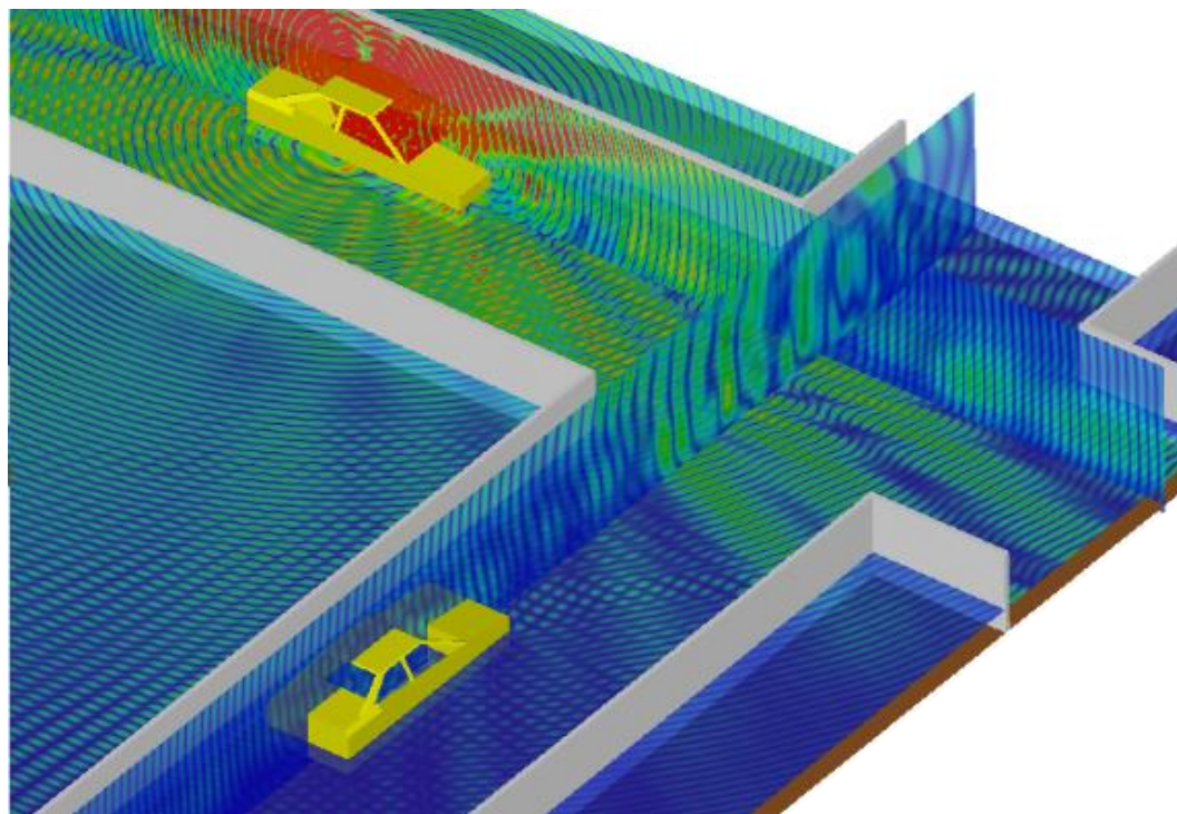
交差点における電界分布
