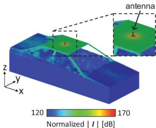
a) 電流分布
