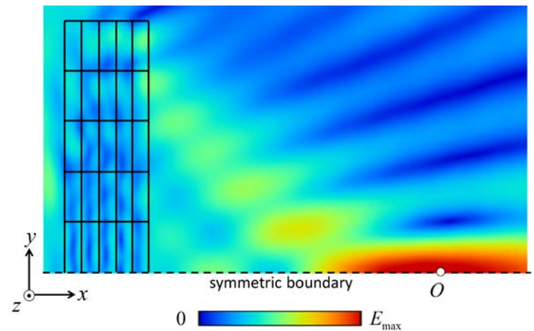
電界分布(5 × 5ブロック, f=30GHz)
