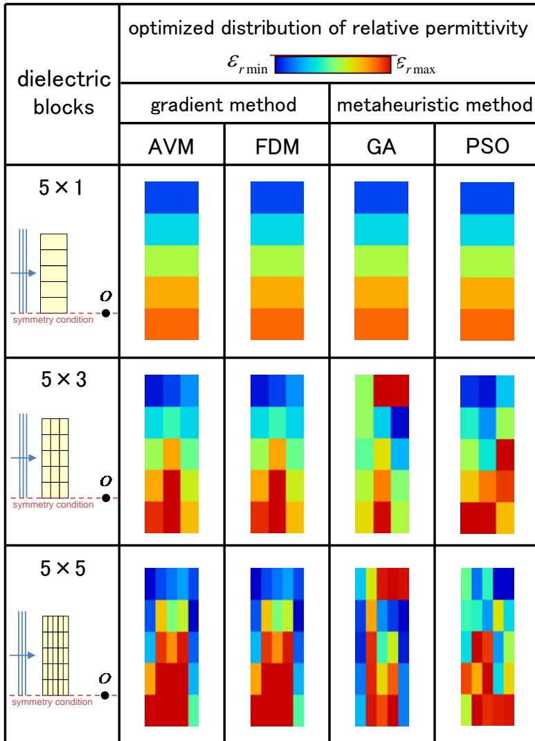
レンズの比誘電率分布比較
