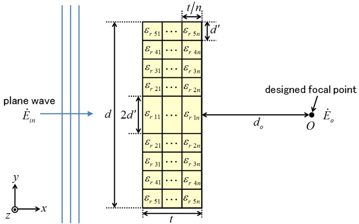
誘電体平面レンズの設計
