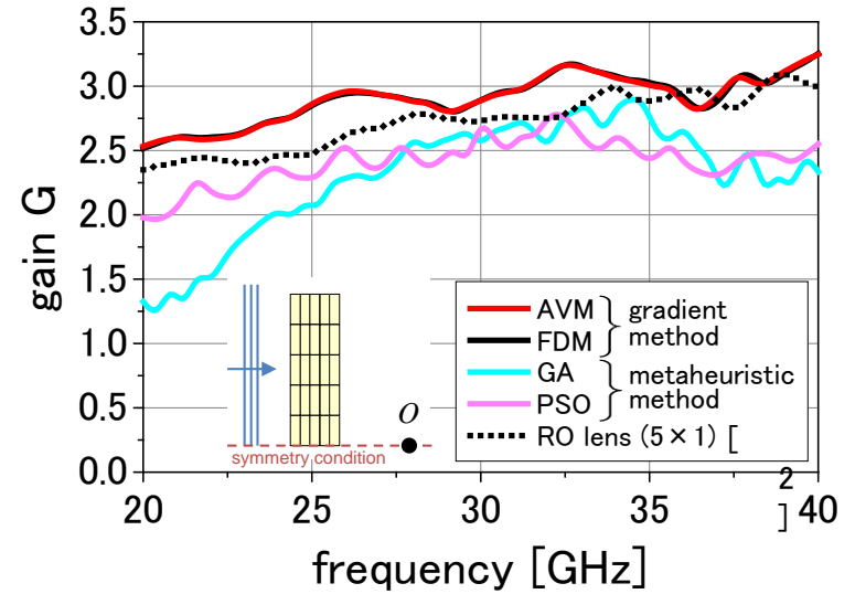
レンズの利得特性比較 (5 × 5ブロック)
