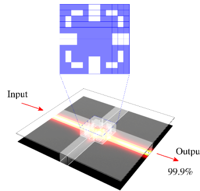
最適化NRD線路交差 (optimized)
