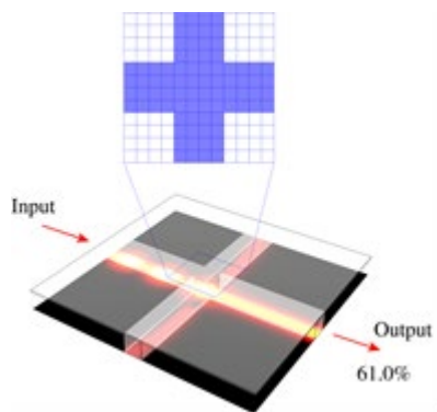
通常のNRD線路交差 (initial)
