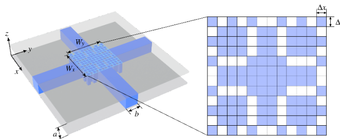
NRD線路交差
