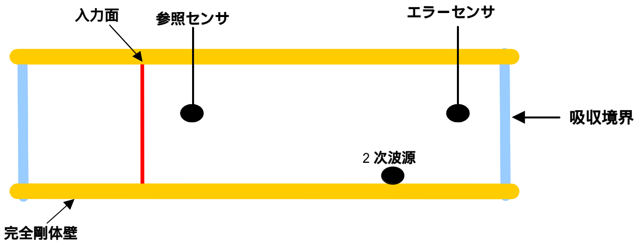
2次元無限長ダクトモデル
