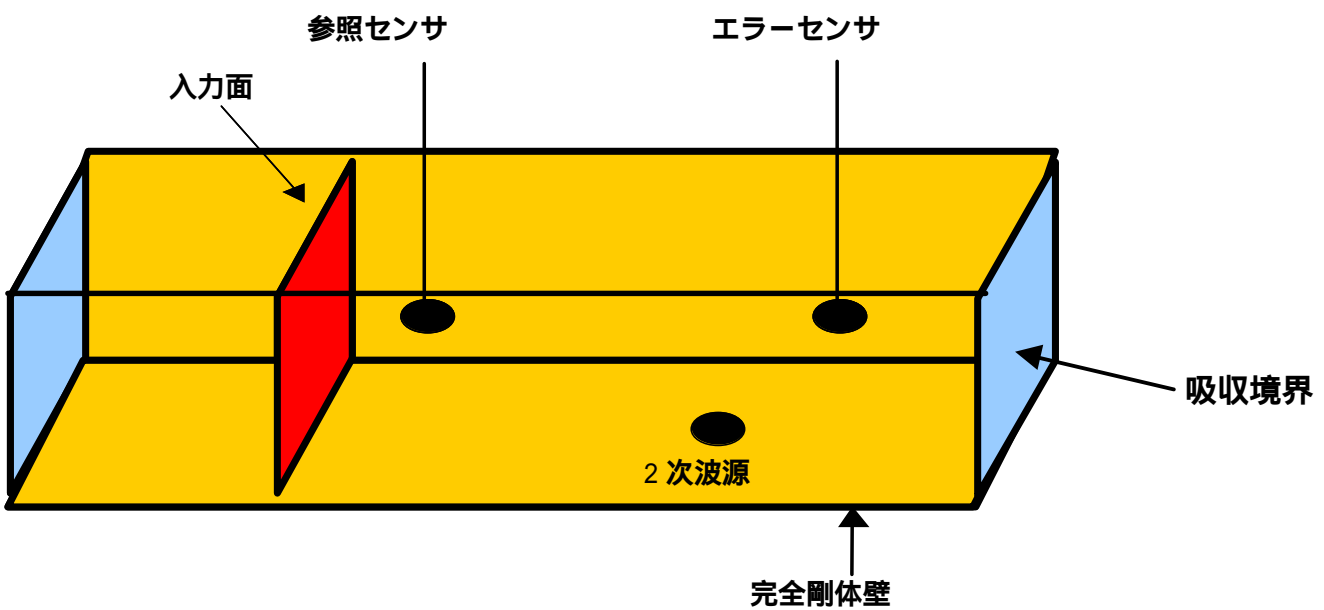
3次元無限長ダクトモデル
