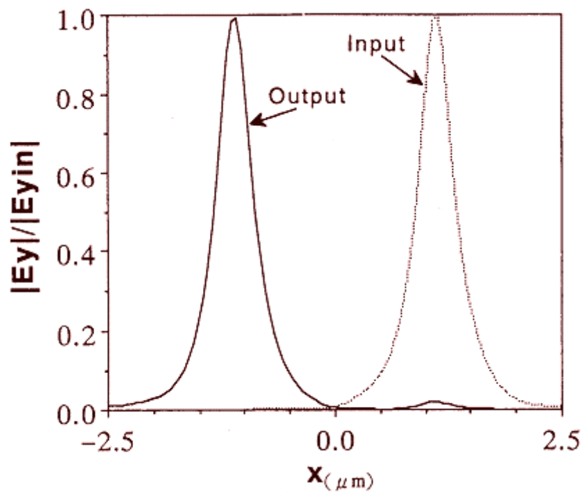
入出力断面の電界成分 E_y の分布
