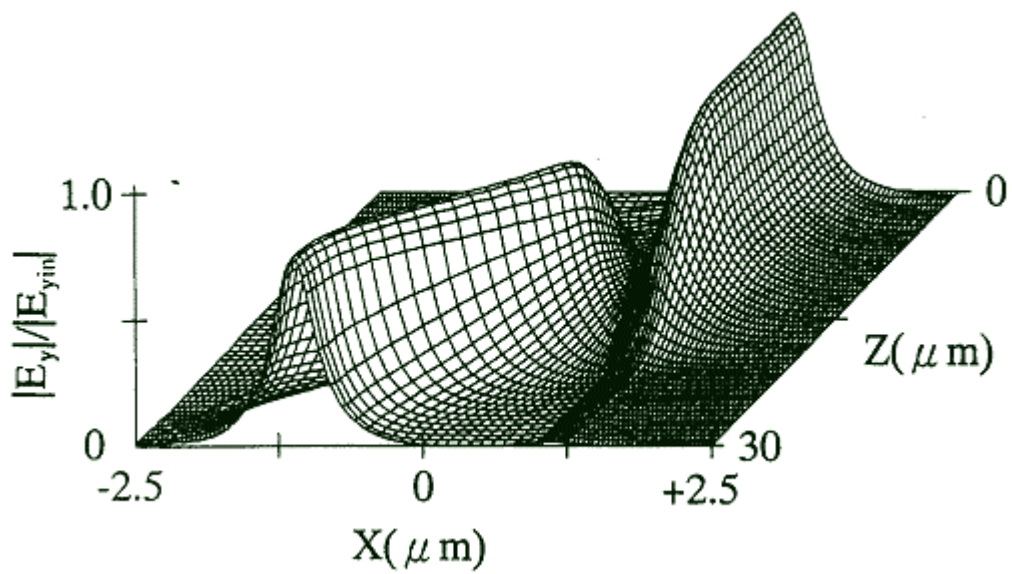
電界成分 E_y の分布
