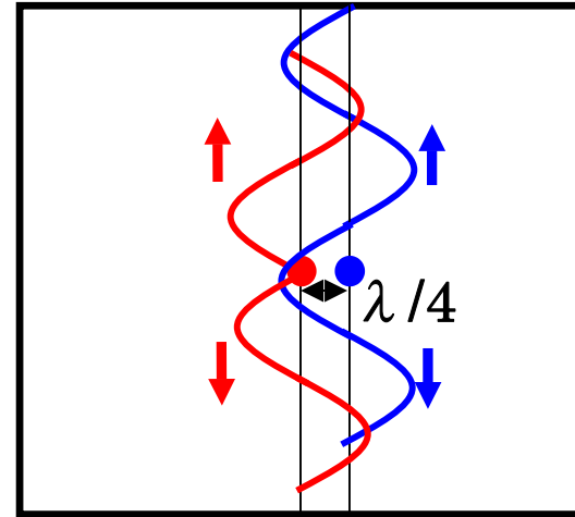
垂直方向の干渉図 (位相差 \psi = \pi/2 )
