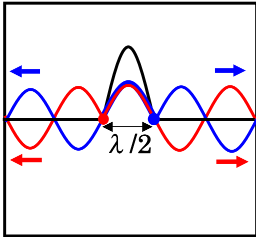
水平方向の干渉図 (位相差 \psi = 0 )
