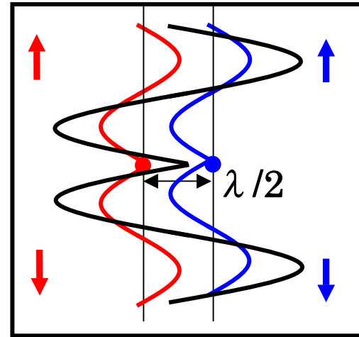
垂直方向の干渉図 (位相差 \psi = 0 )
