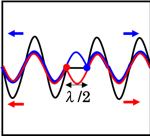
水平方向の干渉図 (位相差 \psi = \pi )
