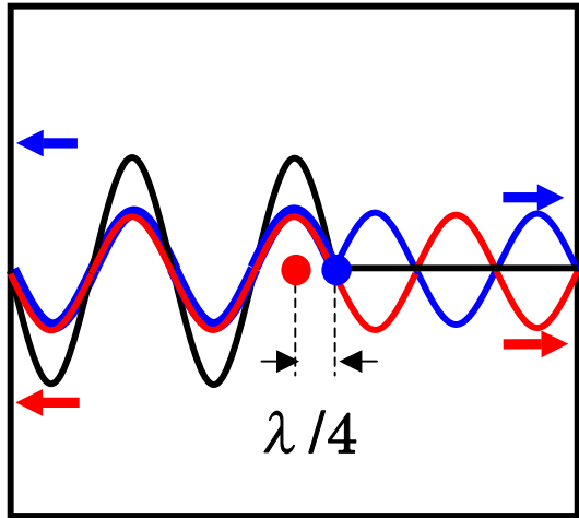
水平方向の干渉図 (位相差 \psi = \pi/2 )
