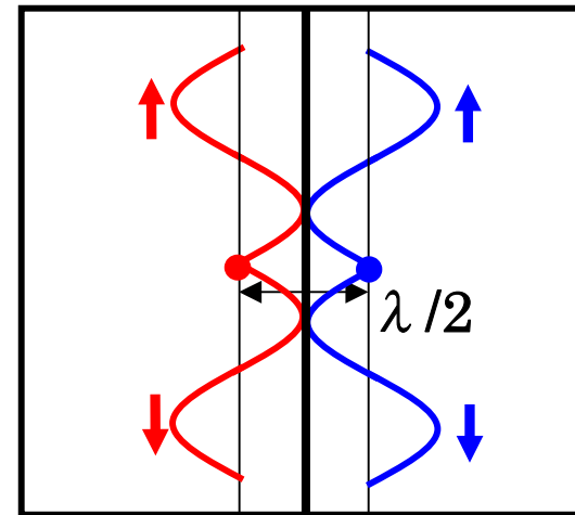
垂直方向の干渉図 (位相差 \psi = \pi )
